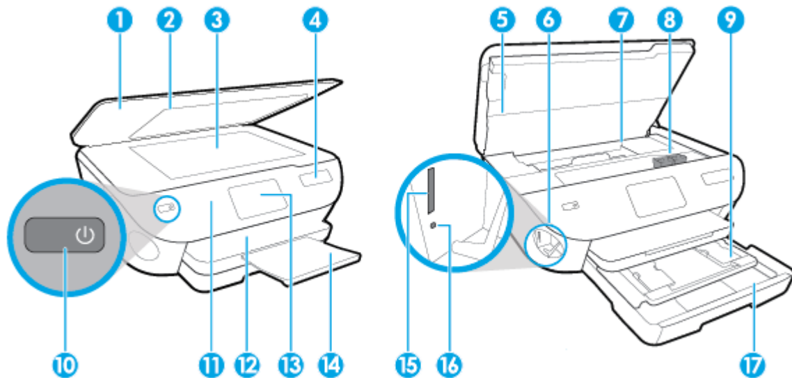
Abbildung 2-1 Ansichten der Vorder- und Oberseite des HP ENVY Photo 7100 All-in-One series
